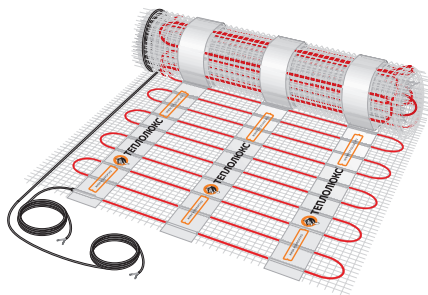
Одножильный мат ТЕПЛОЛЮКС Mini
