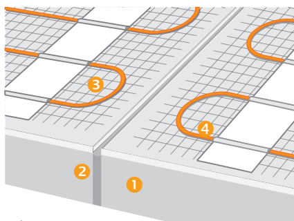
1 – основание 2 – деформационный шов 3, 4 – нагревательные маты
