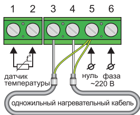
Схема подключения к 2-х проводной электрической сети
